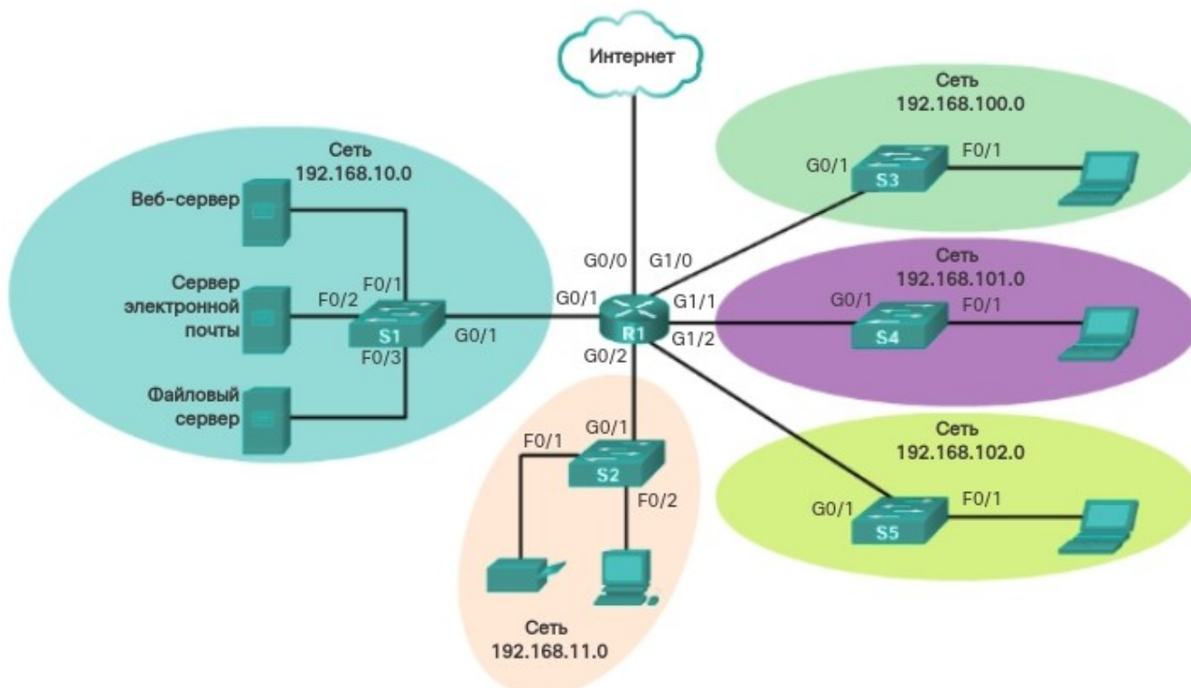
Рисунок 1 – Пример графического представления логической топологии сети
